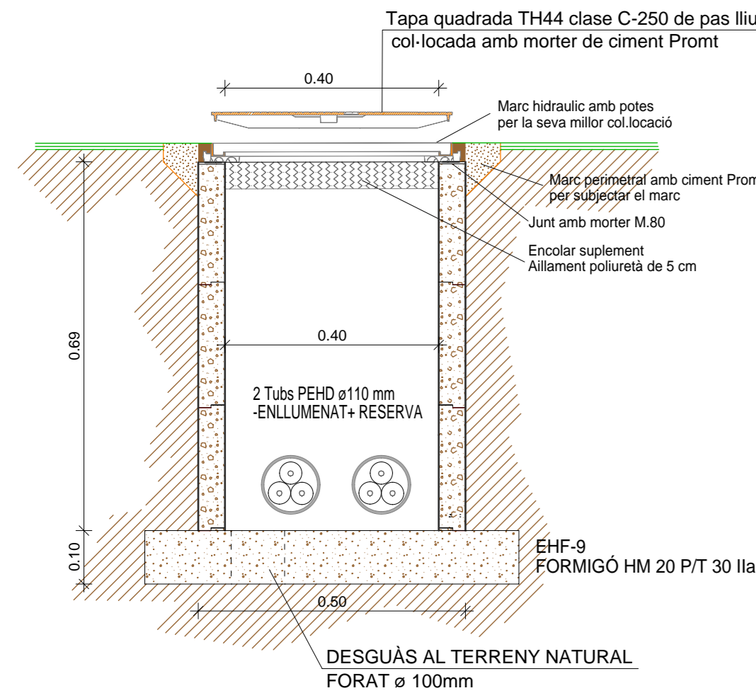
SECCIÓ ARQUETA CONTROL ENLLUMENAT (vorera) IER-25
