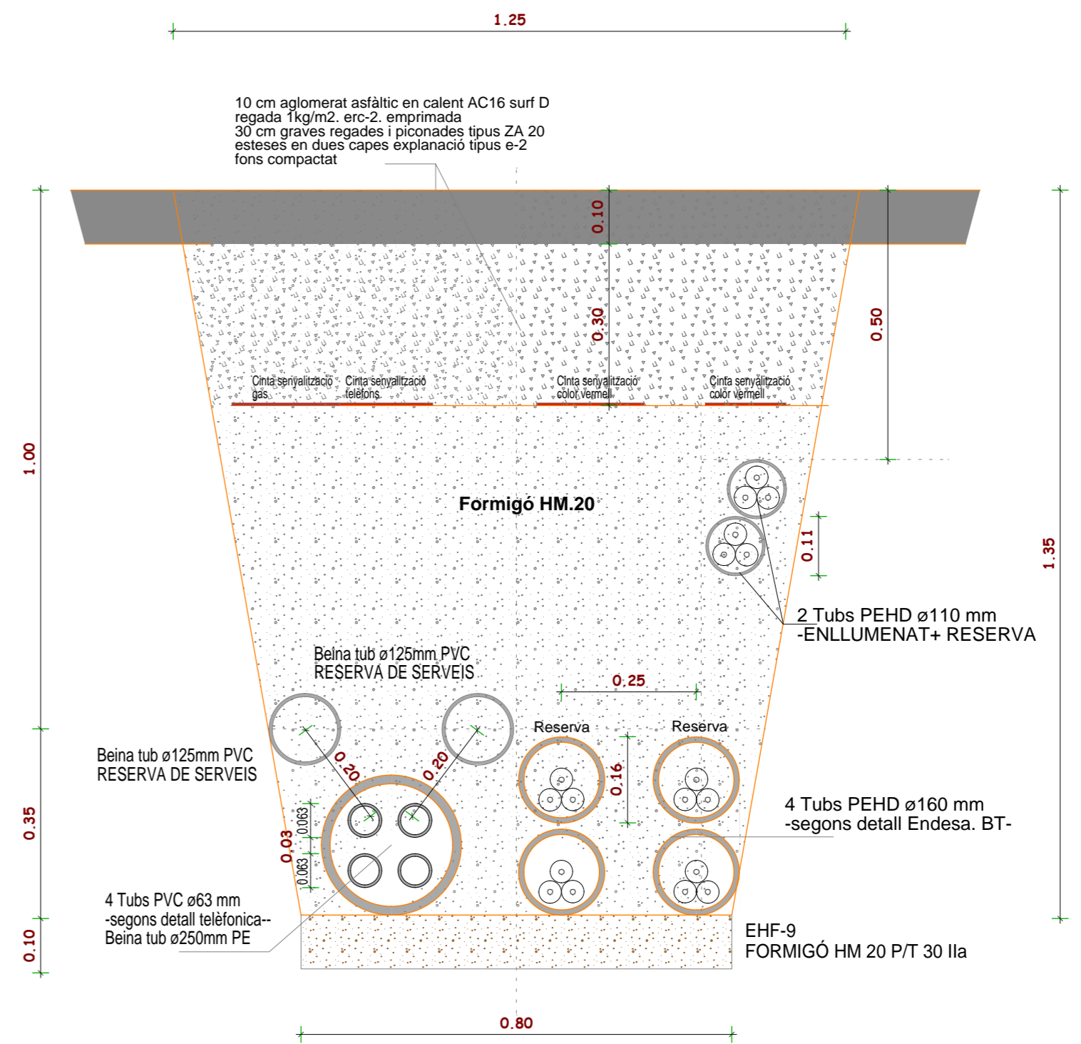
SECCIÓ TRANSVERSAL RASA PAS CARRETERA
