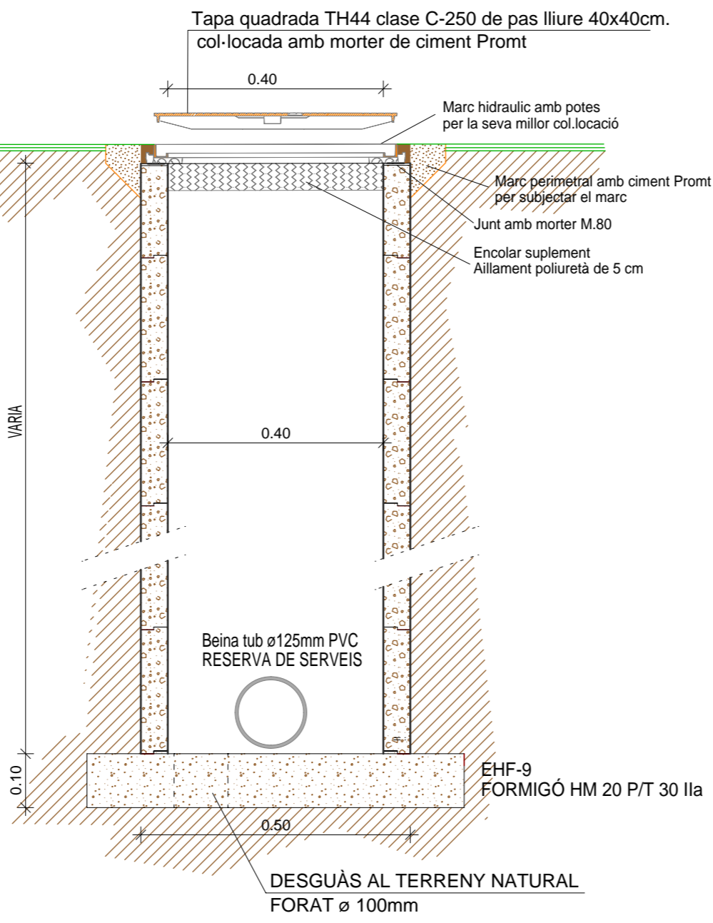
SECCIÓ ARQUETA RESERVA. (vorera) IFA.25
