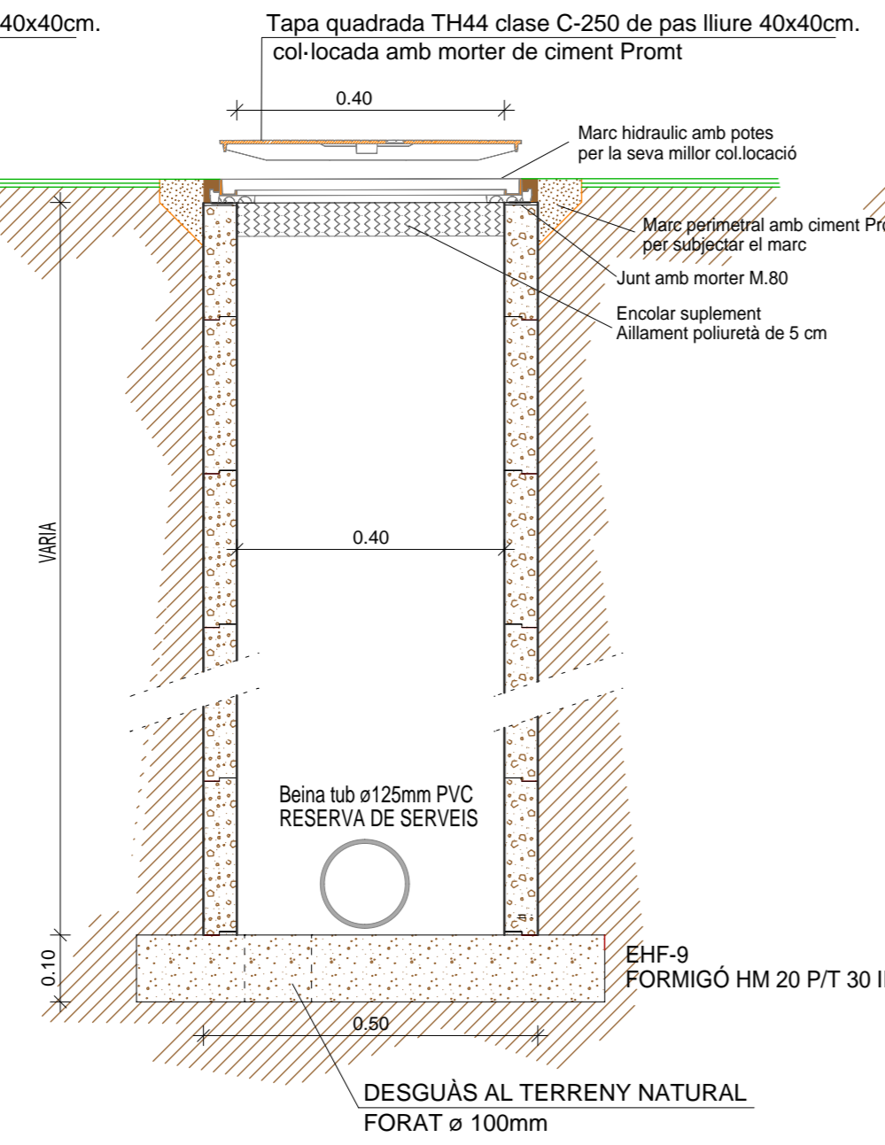
SECCIÓ ARQUETA RESERVA. (vorera) IGL. 25
