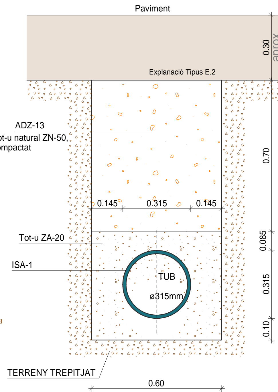
SECCIÓ TIPUS CLAVEGUERAM ISA-8 PE = ISS-45 PE (aigües negres i pluvials)
