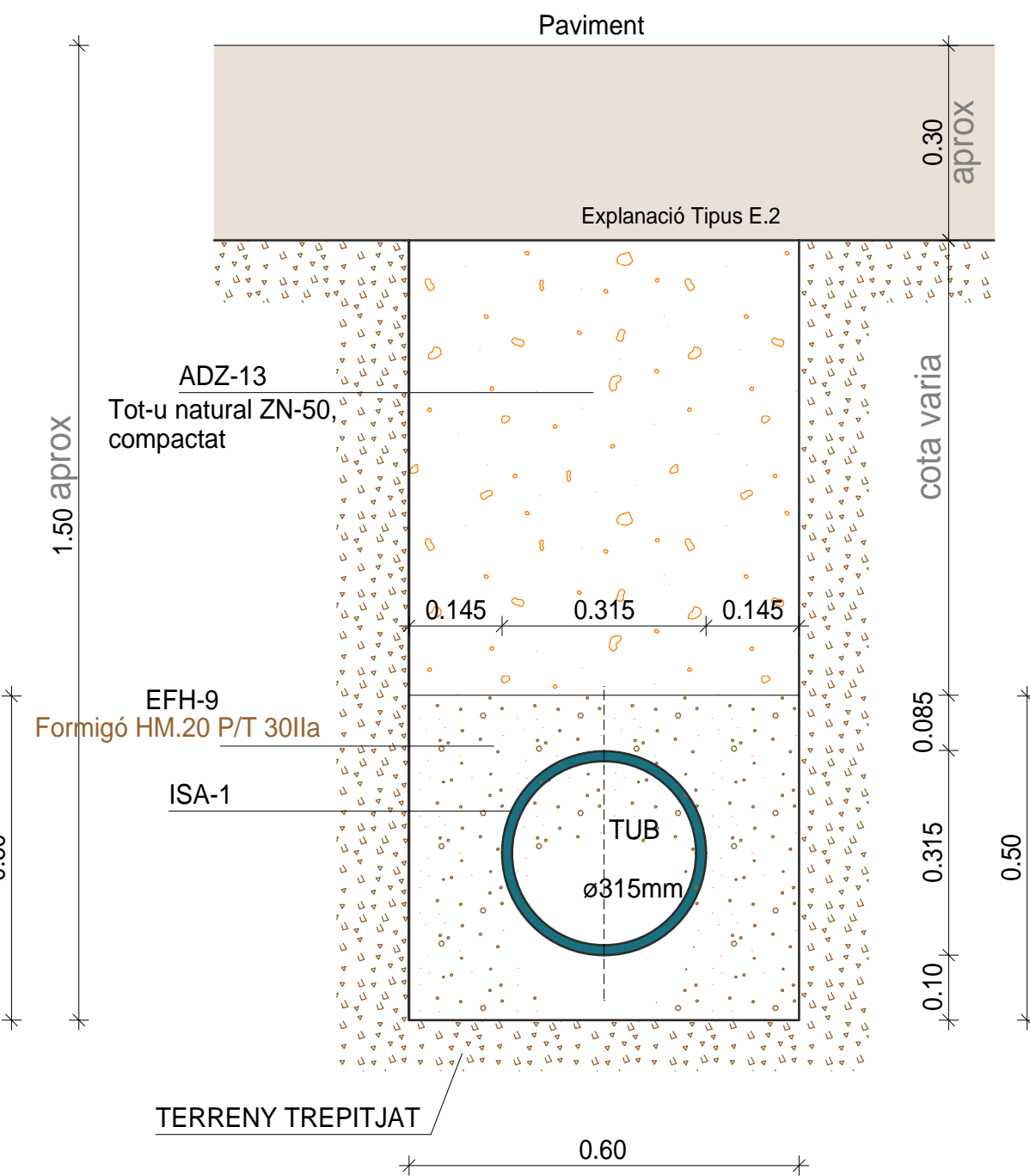
SECCIÓ PEL COSTAT POU, (1.00m de formigó per cada costat del pou) ISA-8 PE = ISS-45 PE (aigües negres i pluvials)
