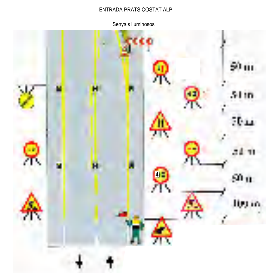
PLÀNOL DESVIAMENT TRÀNSIT OBRES ABANS DE COMENÇAR LES OBRES VERIFICAR AMB L' INFORME TÈCNIC DE LA COMPANYIA TELEFONICA
