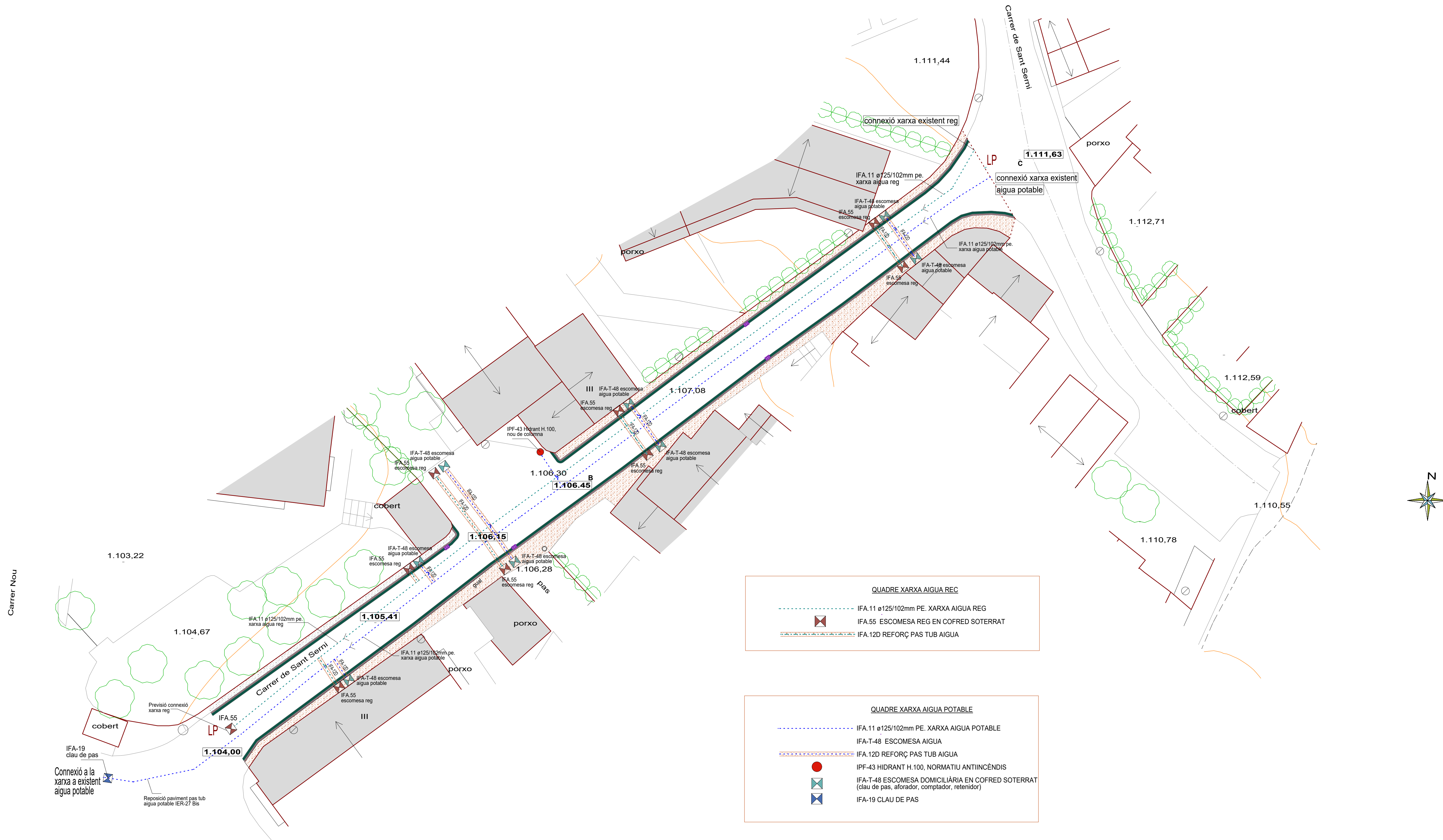
PLÀNOL DE PLANTA -XARXA DE REG- -AIGUA POTABLE- Carrer de Sant Serni
